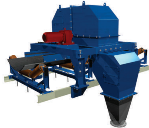
Amostrador tipo Cross Belt
