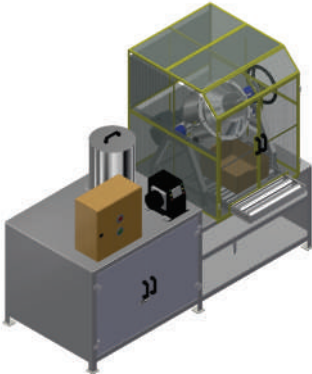
Betoneira de bancada para laboratório
